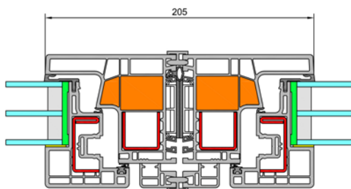
Schnitt Kopplung
